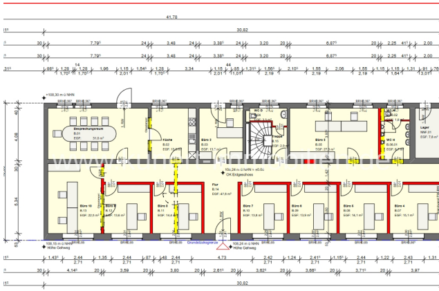
Bürofläche 255.70 m 2
